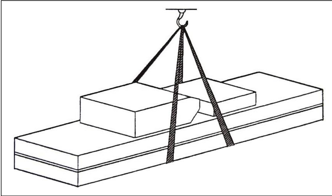
Kuva 2. Pakkauksen nostaminen
