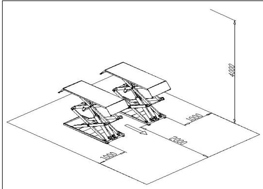
Kuva 13. Asennustilan mitat
