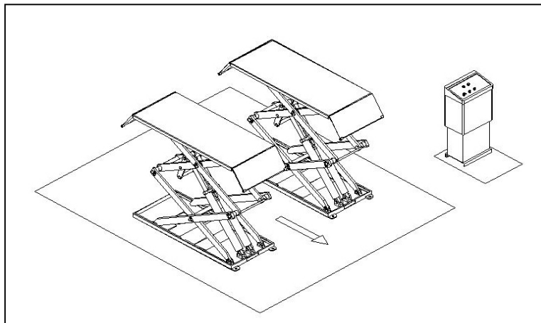
Kuva 6. Nostimen turva-alue
