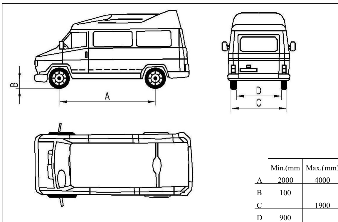
Kuva 5. Ajoneuvon enimmäismitat
