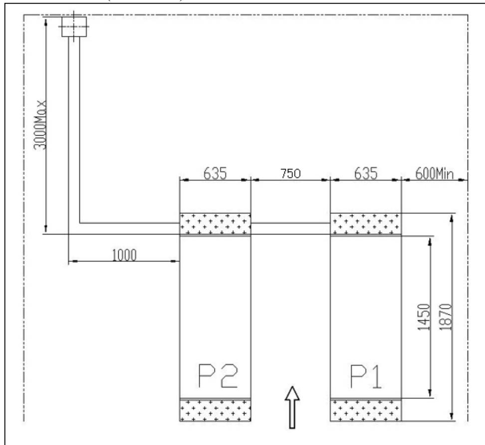
Kuva 4. Kaaviokuva nostimesta (ohjausyksikkö voidaan sijoittaa joko oikealle tai vasemmalle puolelle nostinta)
